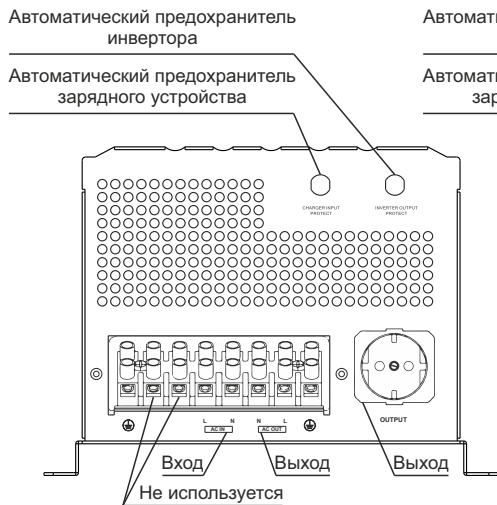
Боковая панель переменного тока (1-3кВт)
