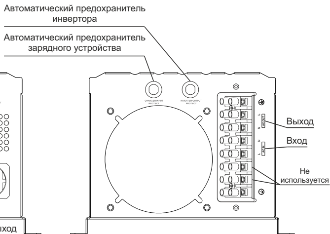
Боковая панель переменного тока (4-6кВт)
