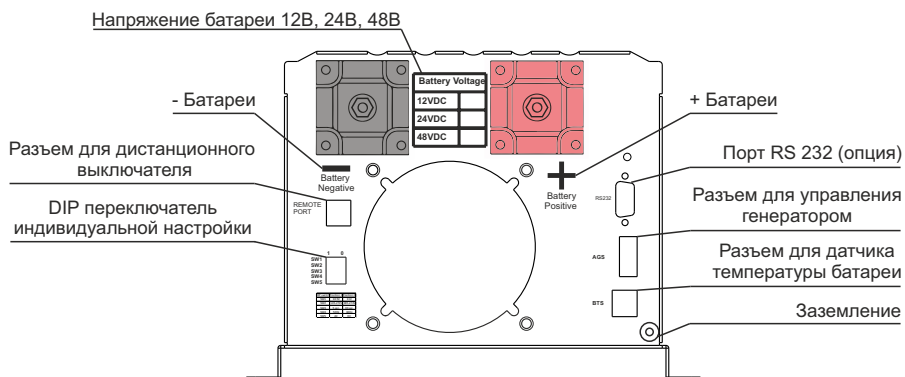
Боковая панель постоянного тока (1-6кВт)
