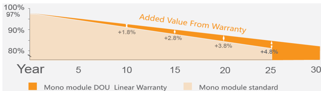
Прогнозируемое сохранение мощности солнечного модуля
