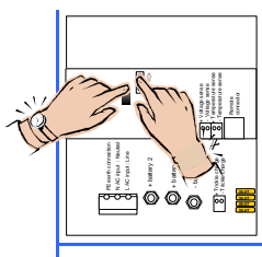
Einstellen des maximalen Konstantstroms
