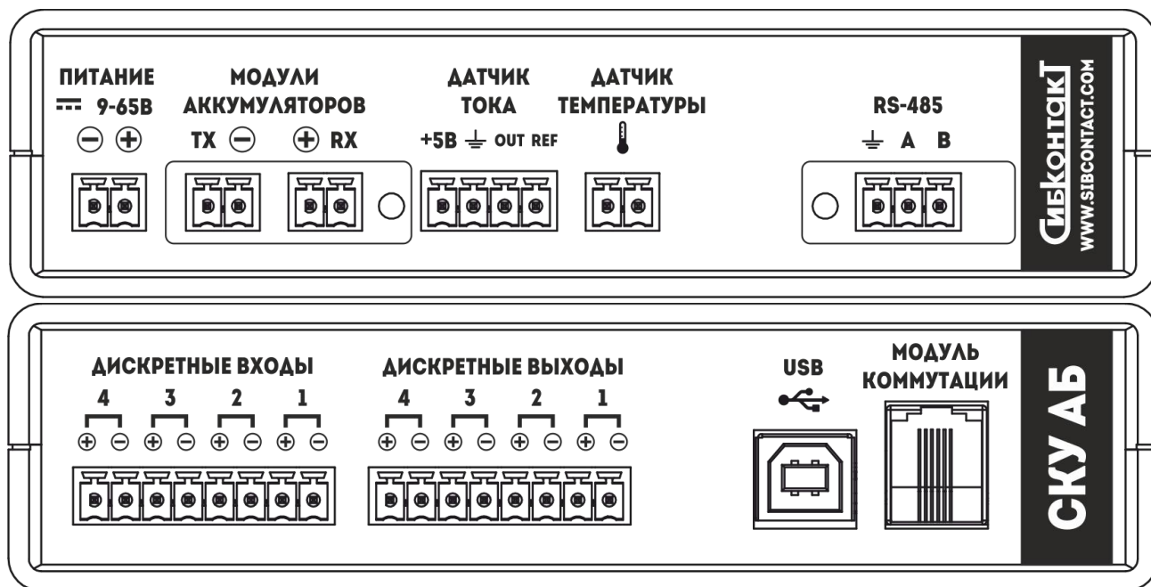
Рис.5. Внешний вид передней и задней панелей МК.
