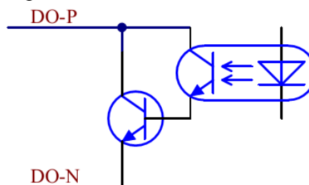
Рис.9. Схема дискретного выхода модуля контроллера.
