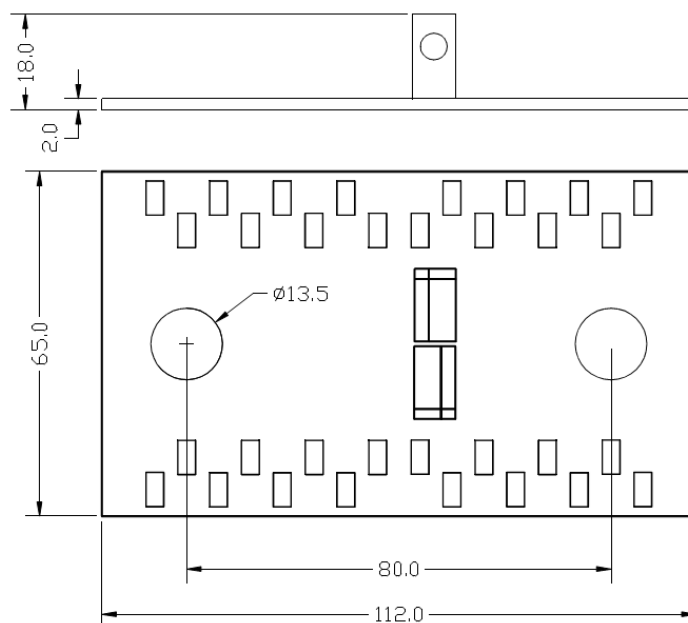
Рис.2. МА с межцентровым расстоянием 80мм.
